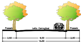
G-1 VIA URBANA LOCAL OU SECUNDARIA VIA SECUNDARIA - LOTEAMENTO FECHADO DECLIVIDADE MAXIMA 12% ESC. 1:100 (*) Somente Autorizado com Diretriz Municipal.
