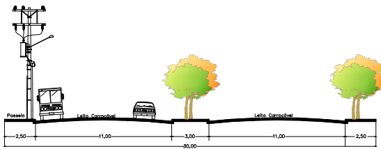
G-1 VIA URBANA LOCAL OU SECUNDARIA VIA SECUNDARIA - LOTEAMENTO FECHADO DECLIVIDADE MAXIMA 12% ESC. 1:100 (*) Somente Autorizado com Diretriz Municipal.
