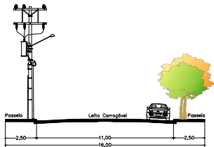
G-2 VIA URBANA COLETOIRA TIPO II VIA LOTEAMENTO FECHADO DECLIVIDADE MAXIMA 12% ESC. 1:100
